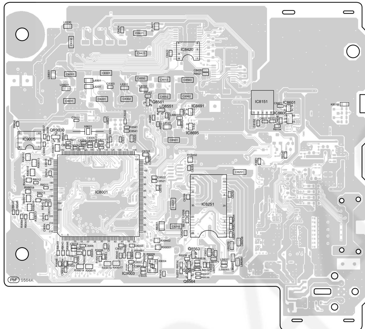
A DVD MODULE P.C.B. (REPX0620F-M)
