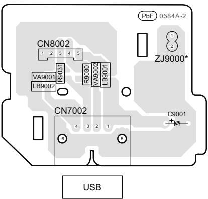
J USB P.C.B. (REPX0658F)
