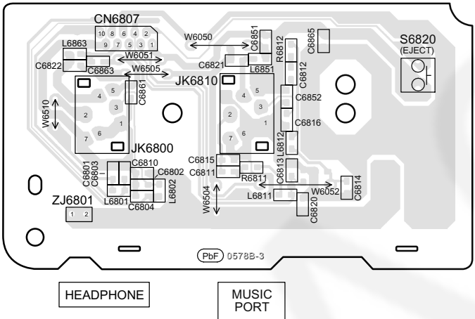
G MUSIC PORT P.C.B. (REPX0671B)
