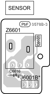
H REMOTE SENSOR P.C.B. (REPX0671B)
