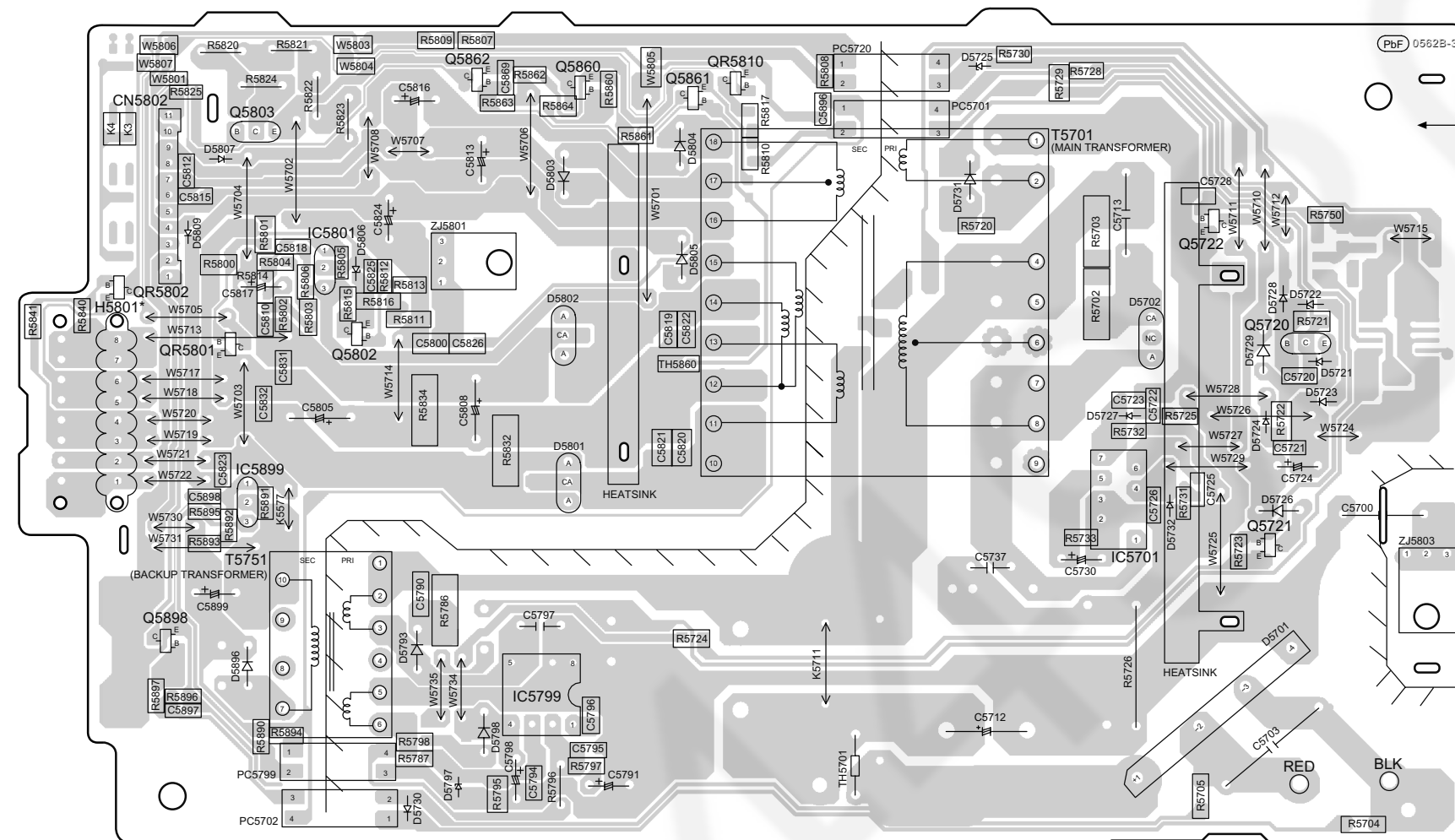
N SMPS P.C.B. (REPX0676A)
