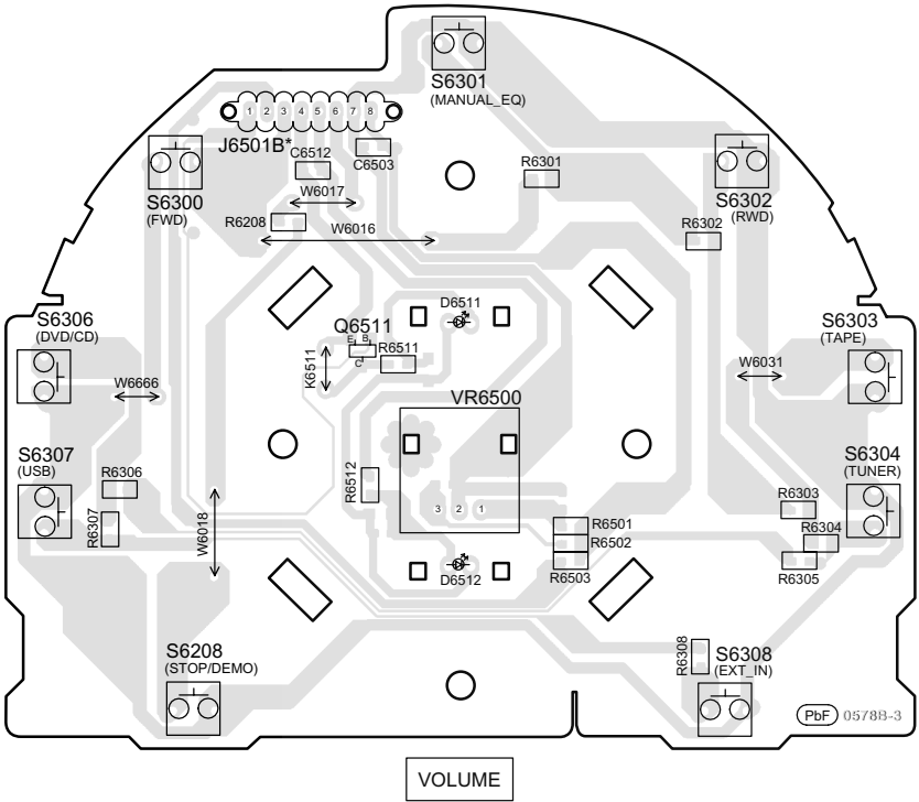
F TACT SWITCH P.C.B. (REPX0671B)
